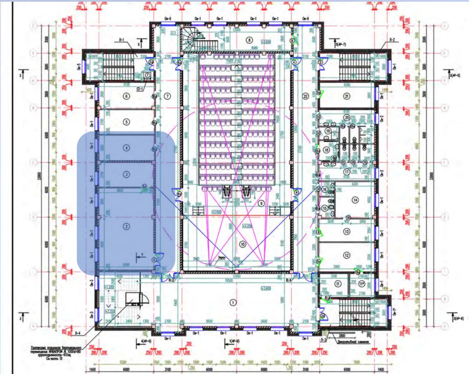
План 2 этажа
